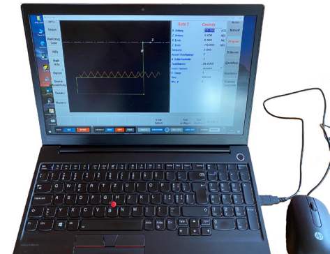
Offline-Programmiersystem mit DXF-Konverter
